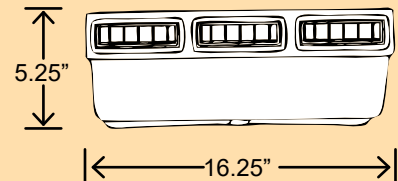
Mini Slim Line Dimension Detail
